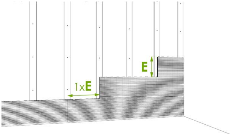
Abb. 4g E = Elementbreite, Beachte Versatz Längsstöße
