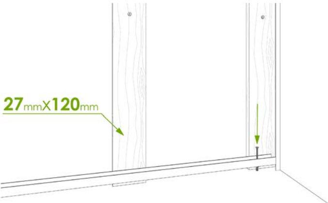
Abb. 4d Detail: Vorschlag Abschlussvariante zum Boden – Bodenprofil
