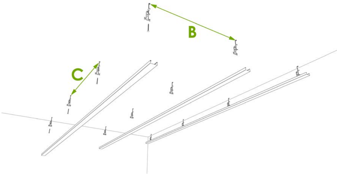
Abb. 1a: Erste Unterkonstruktion mit Stahlblechprofilen
