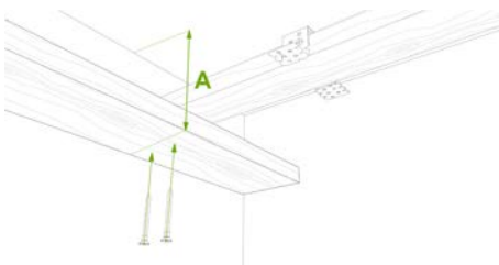
Detail 2c Befestigung mit 2 Schrauben, Abhänghöhe A = Abstand von Rohdecke zu Unterkante der zweiten Unterkonstruktion
