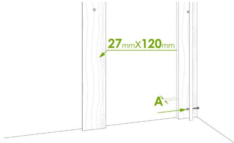
Abb. 4c: Montage Wandanschlussprofil A = Abstand von Wand zu Außenkante Unterkonstruktion
