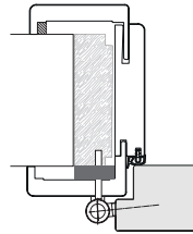
■ Reno-System KUNEXPlus: auf Holzstock
