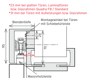
■ 1b Blende flächenbündig Verkleidungsbreite 50 mm (nicht in Verbindung mit Seilzug möglich)
