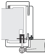
■ Reno-System KUNEXPlus: auf Stahlzarge
