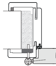
■ Reno-System KUNEXPlus: auf Holzstock
