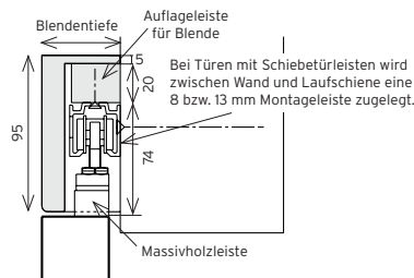
■ 1b Blende flächenbündig (nicht in Verbindung mit Seilzug möglich)
