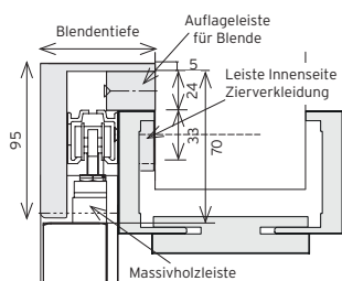
■ 3b Blende flächenbündig mit Anschlagpfosten flächenbündig
