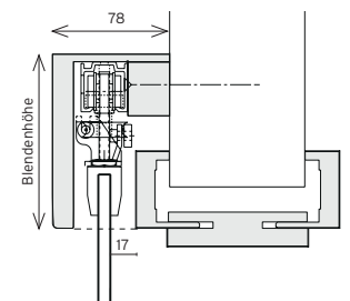
■ 2d 2-flügelig mit Seilzug Verkleidungsbreite 50 mm
