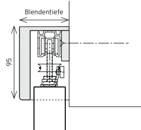
■ 1c 2-flügelig mit Seilzug (nicht in Verbindung mit bündiger Blende möglich)
