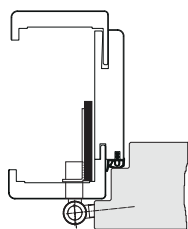
■ VARIANTE: Einsatz auf Einfachfalz-Zarge (Schallschutz 47 dB nur in Verbindung mit Doppelfalz-Zarge möglich)
