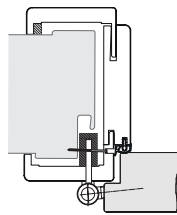
■ Reno-System KUNEXPlus: auf Stahlzarge
