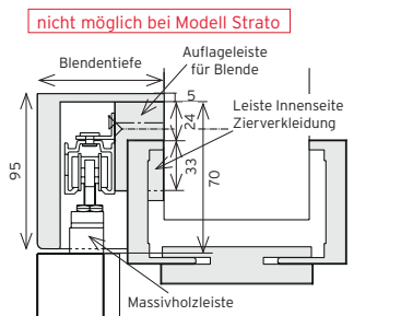
■ 1b Blende flächenbündig Verkleidungsbreite 75 mm (nicht in Verbindung mit Seilzug möglich)
