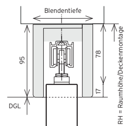
■ 2 Geschoßhoch Bodenluft bei Standard-Laufschiene ca. 6 mm
