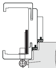
■ STANDARD: auf Mauerwerk
