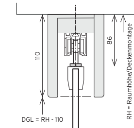
■ 1b Geschoßhoch Bodenluft bei Standard-Laufschiene ca. 9 mm
