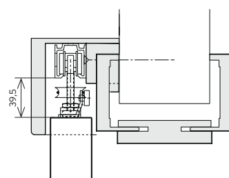
■ 1c 2-flügelig mit Seilzug Verkleidungsbreite 75 mm (nicht in Verbindung mit bündiger Blende möglich)
