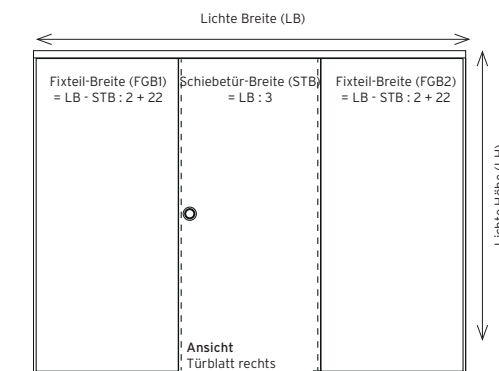
■ 2 Ausführung mit 2 Fixteilen (max. Wandöffnung 3534 x 2640 mm)
