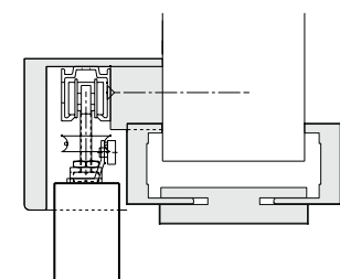
■ 1c 2-flügelig mit Seilzug Verkleidungsbreite 50 mm (nicht in Verbindung mit bündiger Blende möglich)
