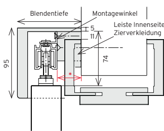
■ 1a Standard Verkleidungsbreite 75 mm
