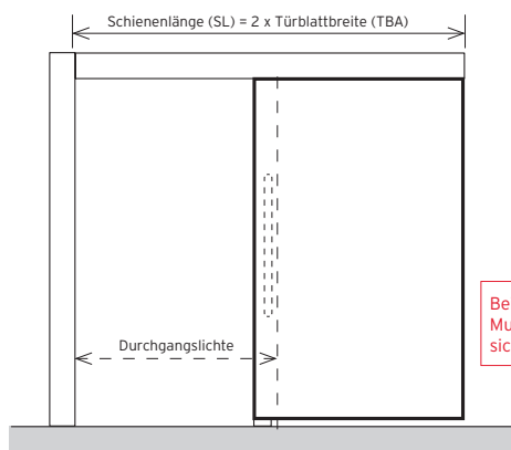
Abbildung: Links schließend = rechtes Türblatt
