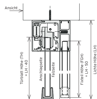
■ Metall-Abdeckblende / Deckenmontage (Wandmontage nur bedingt möglich)
