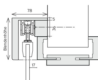
■ 2b Standard Verkleidungsbreite 50 mm
