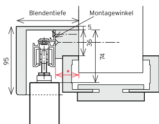
■ 1a Standard Verkleidungsbreite 50 mm
