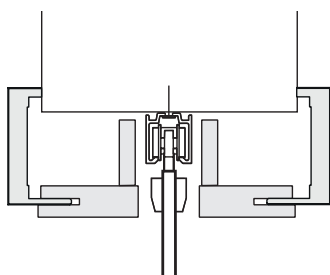
■ 1 Standard ohne Schiebetür-Kastensystem
