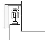
Holz-Schiebetürblatt OHNE FERTIGZARGE
