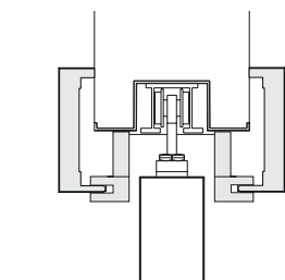
■ 1b Schiebetür-Kastensystem Einbaukasten bauseits
