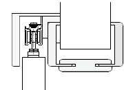
Holz-Schiebetürelement MIT FERTIGZARGE
