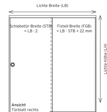
■ 1 Ausführung mit 1 Fixteil (max. Wandöffnung 2356 x 2640 mm)
