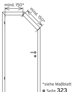
■ Türelement mit Schräge
