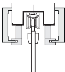
■ 1 Schiebetür-Kastensystem Einbaukasten bauseits
