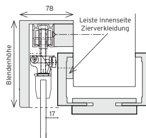
■ 2c 2-flügelig mit Seilzug Verkleidungsbreite 75 mm
